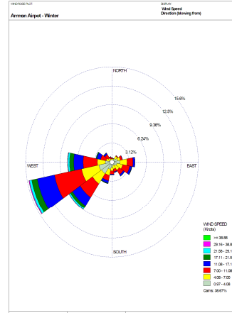
وردة الرياح لمطار عمان المدني خلال الفترة (1991-2020)
